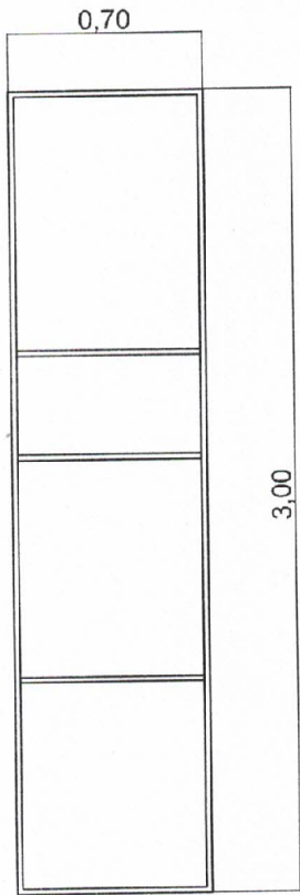
01 VISTA SUPERIOR ARMÁRIO ESCALA 1:50
