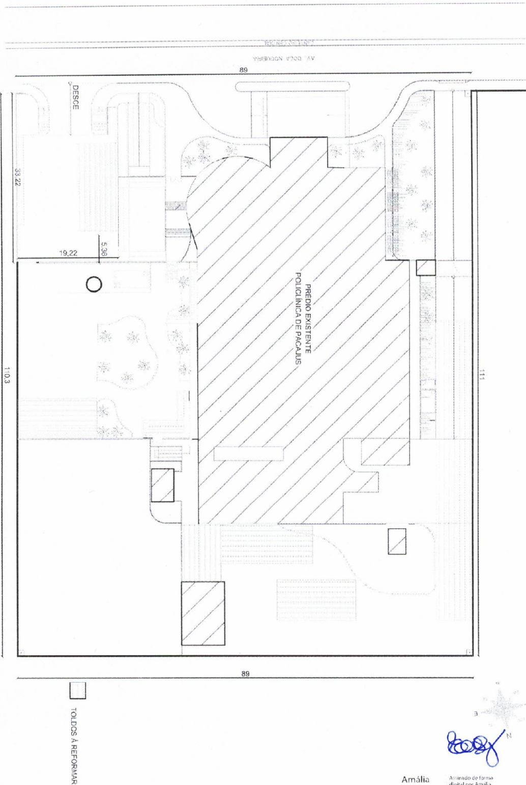
01 PLANTA DE REFORMA DE TOLDOS DO ESTACIONAMENTO ESCALA 1:500
